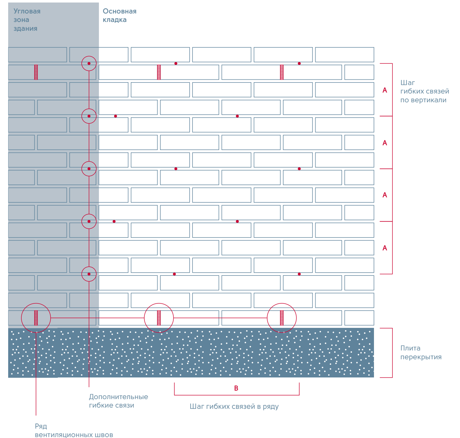
Схема 3. Пример привязки шага установки связей к раскладке лицевого кирпича.
