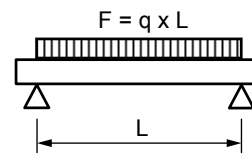
Схема нагружения 3
