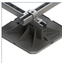
Узел крепления
