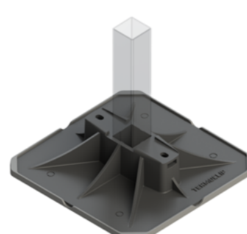
Опора кровельная 335 B50
