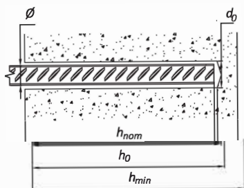
АРМАТУРНЫЙ СТЕРЖЕНЬ В КАЧЕСТВЕ АРМИРОВКИ КОНСТРУКЦИИ
