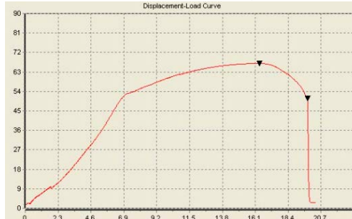
10133-023 SCA M12x250 66,9 кН
