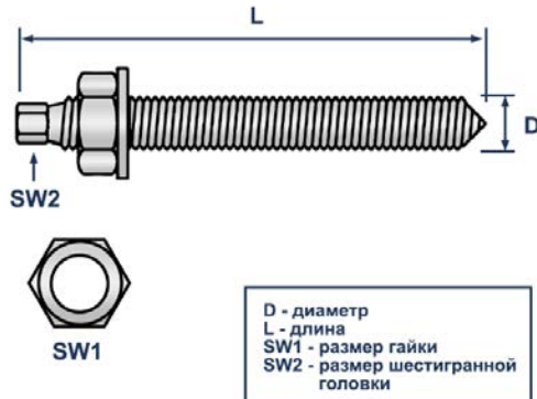
Шпилька анкерная с гайкой и шайбой
