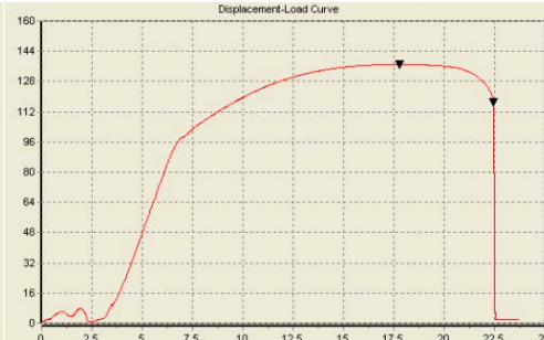
10136-023 SCA M16x250 136,6 кН
