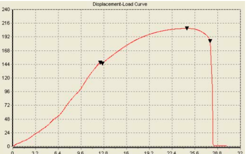
11040-023 SCA M20x245 206,8 кН
