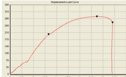
10141-023 SCA M24x300 290,5 кН
