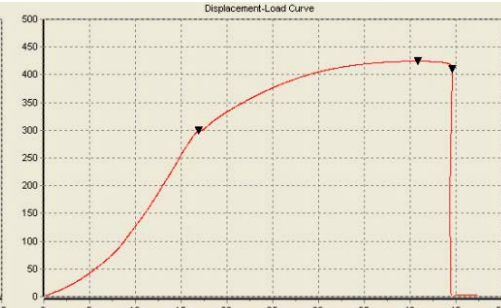
11041-023 SCA M30x400 424,3 кН
