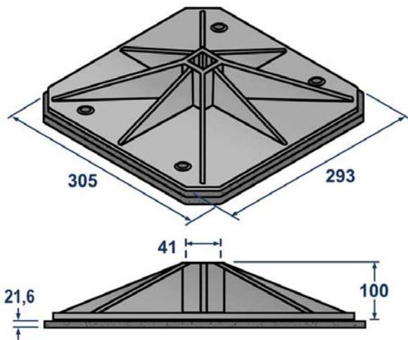
Опора кровельная с антивибрационным ковриком
