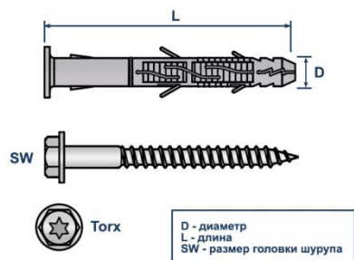
Дюбель фасадный с шестигранным шурупом с прессшайбой
