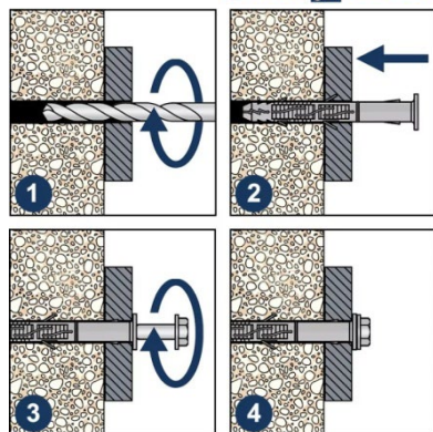
Дюбель фасадный с шестигранным шурупом с прессшайбой
