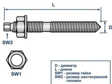
Шпилька анкерная с гайкой и шайбой
